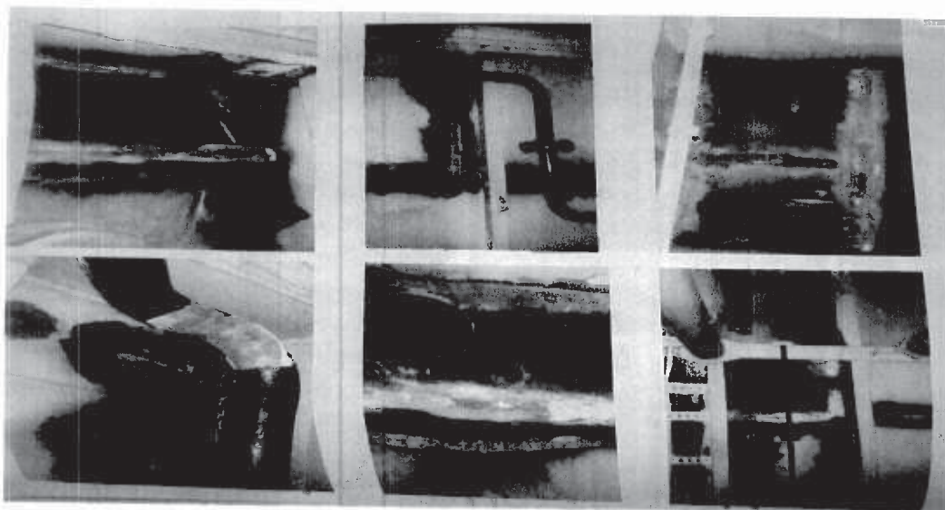
Fuente: Informe Pericial - Perito Maquinaria Naval Pablo Puello- Siniestro Marítimo de Arribada Forzosa de la Motonave "BALBOA EXPLORER" - Folio 94
